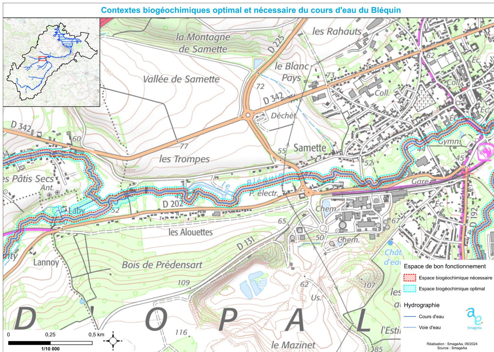
Figure 13 : Exemple des contextes biogéochimiques sur un tronçon du Bléquin
