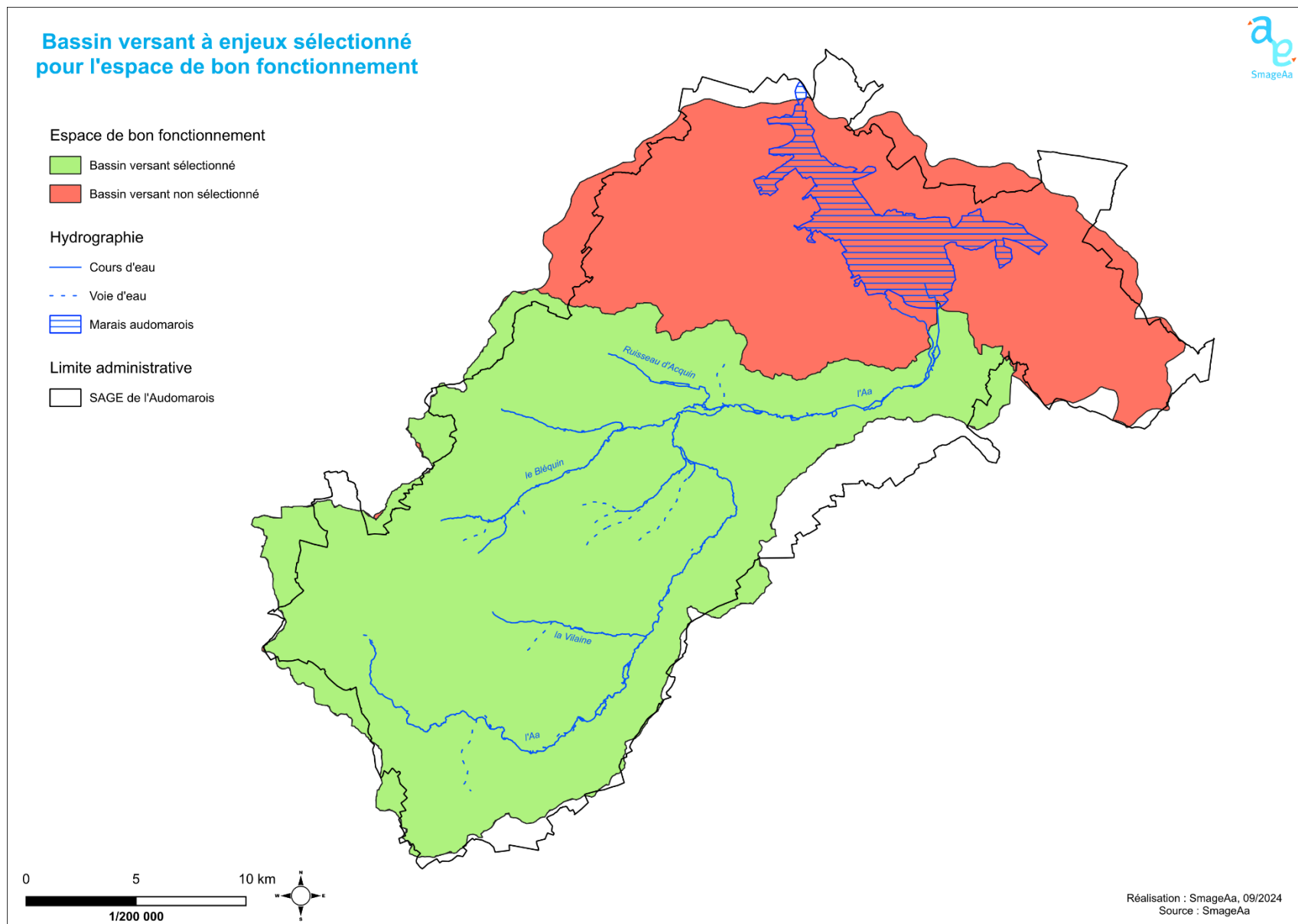
Figure 2 : Cartographie des sous bassins versants du SAGE Audomarois
