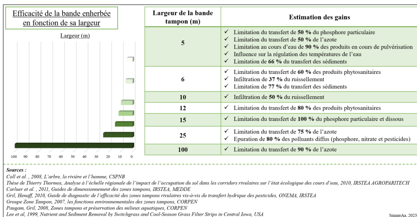
Figure 12 : Figure récapitulative des gains apportés en fonction de la largeur de la bande enherbée
