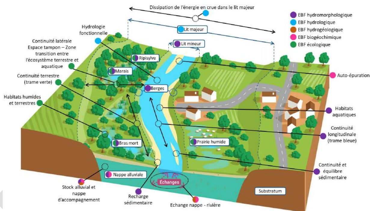
Figure 7 : Schéma explicite des caractéristiques de l'espace de bon fonctionnement, OFB
