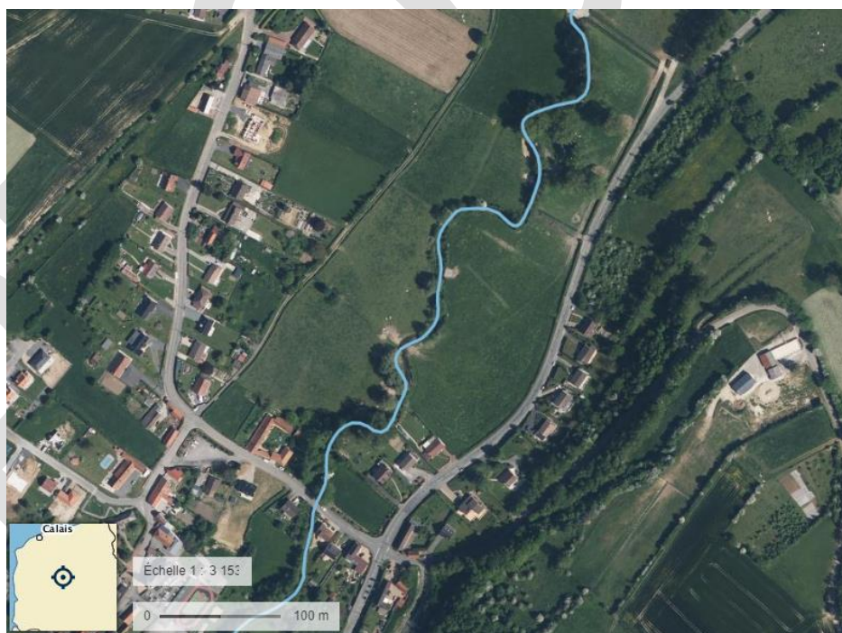
Figure 4 : Photographie aérienne du cours d'eau du Bléquin
