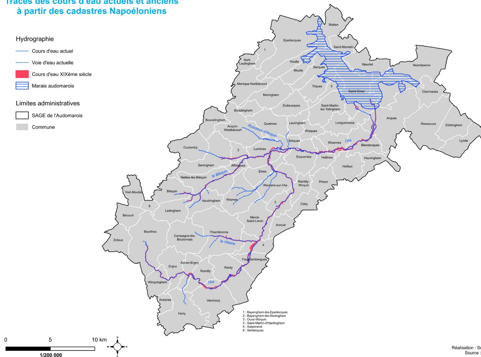
Figure 6 : Cartographie du tracé du cours d'eau à l'époque Napoléonienne et actuelle
