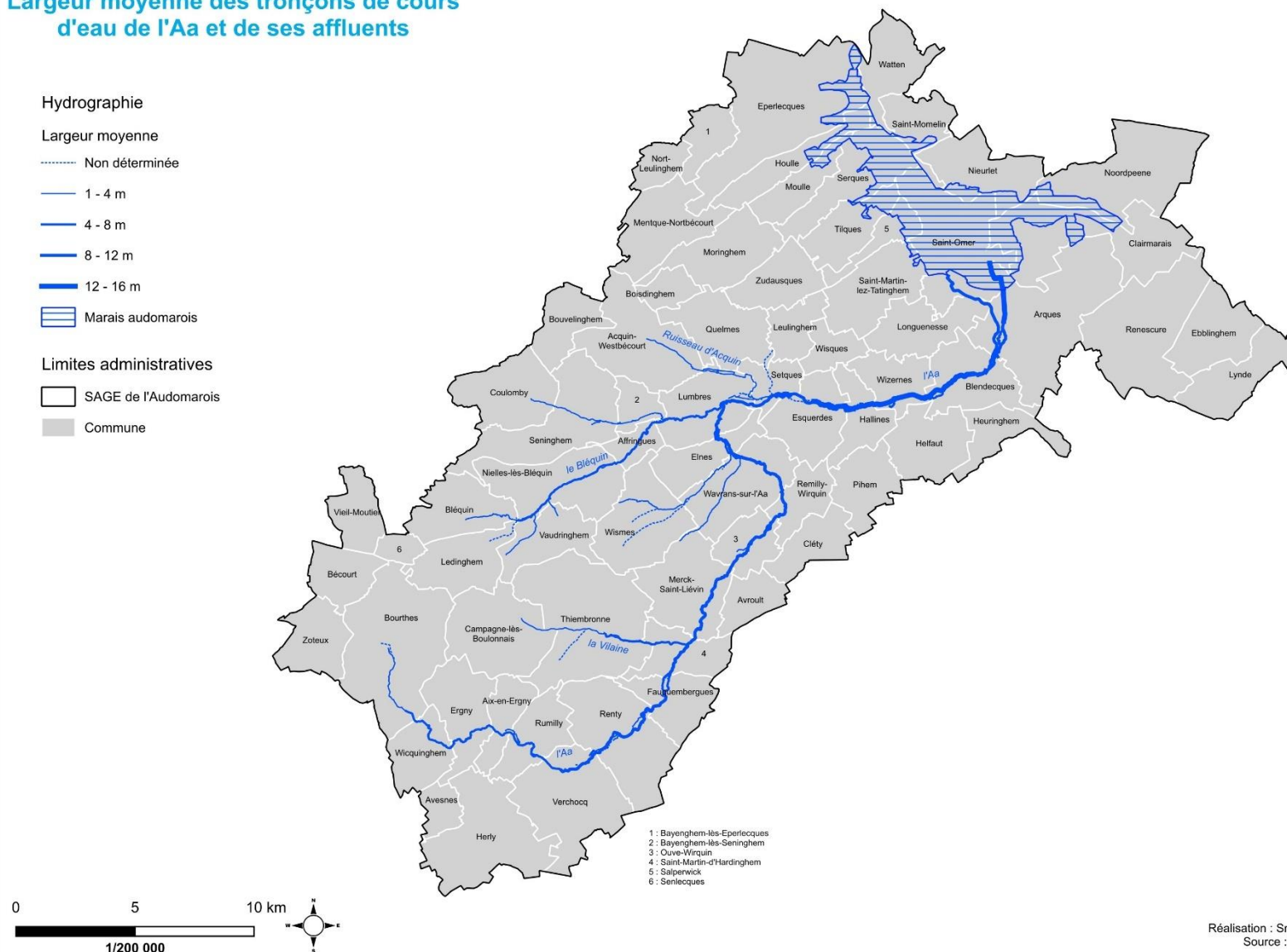
Figure 3 : Cartographie représentant la largeur des tronçons hydrographiques sur la vallée de l'Aa
