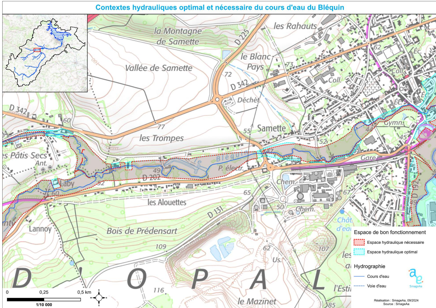
Figure 11 : Exemple des contextes hydrauliques sur un tronçon du Bléquin
