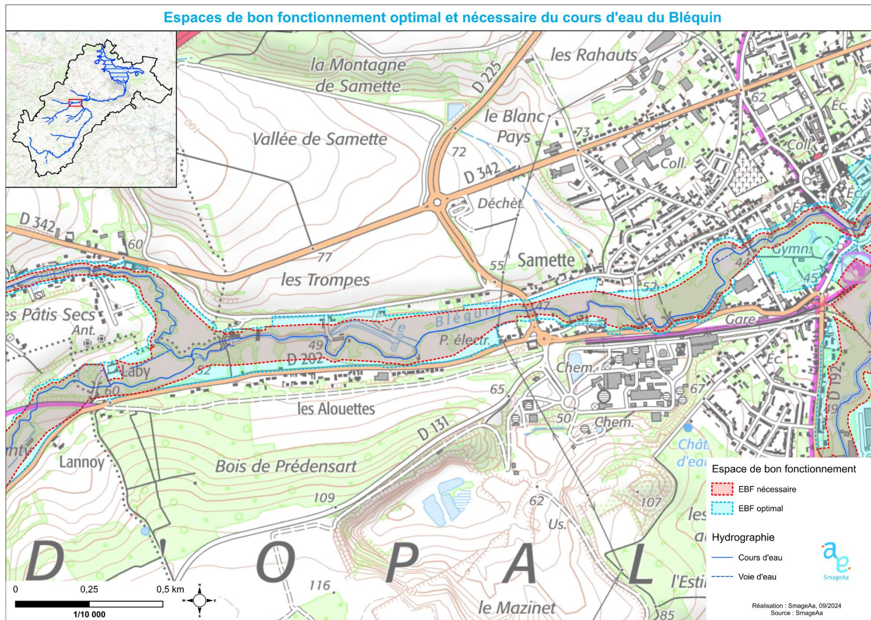
Figure 16 : Exemple d'espaces de bon fonctionnement optimal et nécessaire sur un tronçon du Bléquin
