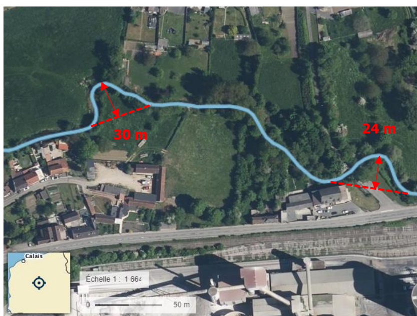
Figure 8 : Exemple de mesures d'amplitudes des méandres sur une photographie aérienne du Bléquin
